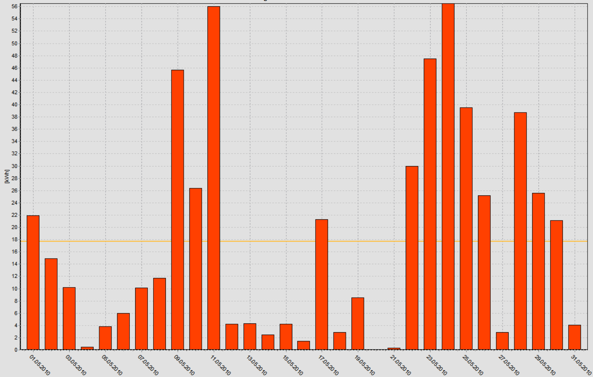
Ertrag 01.05.2010 - 31.05.2010
