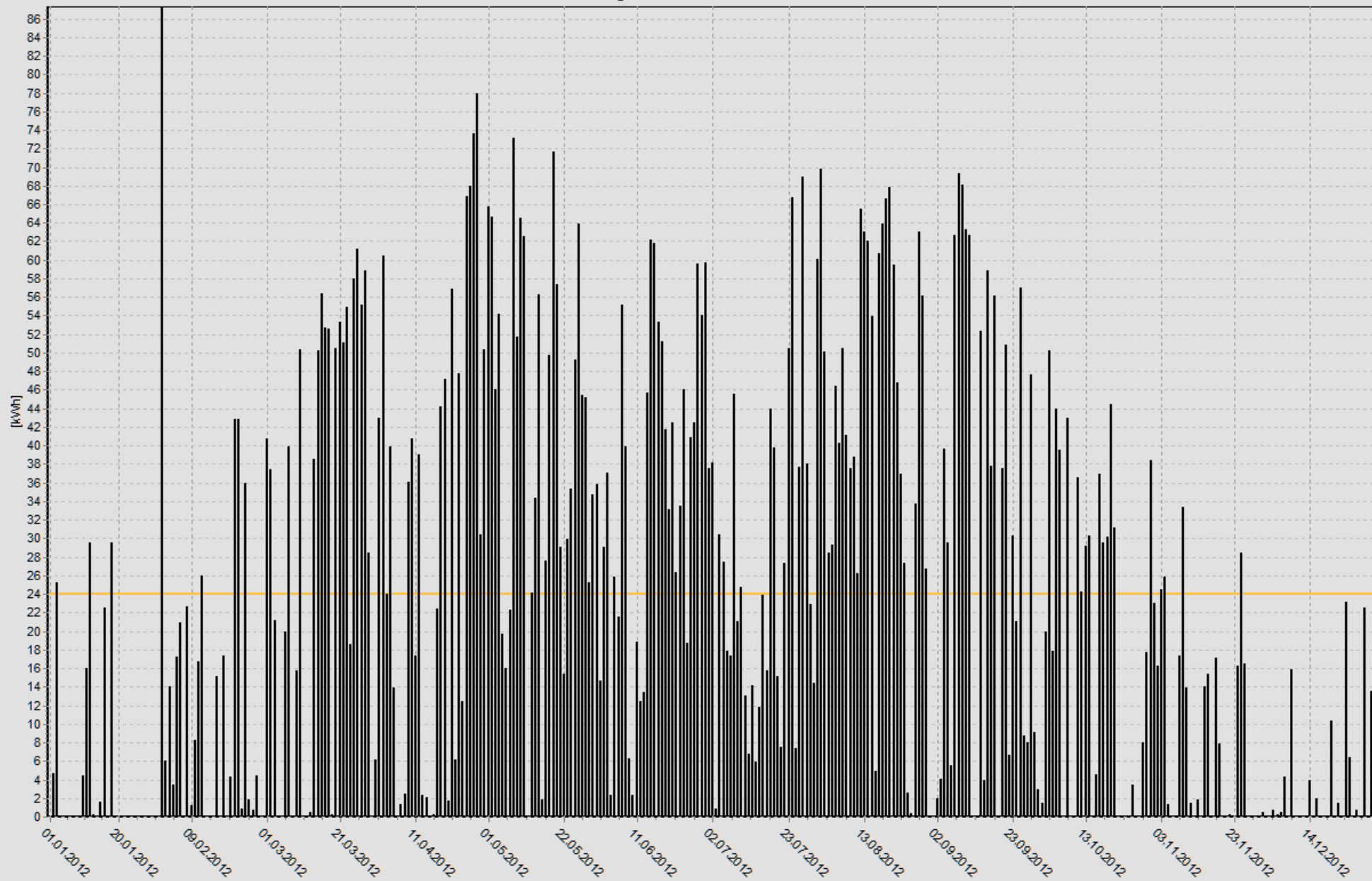
Ertrag 01.01.2012 - 31.12.2012
